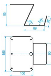
Hanger AK-AF5S
