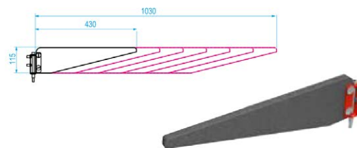
Boxes separator
