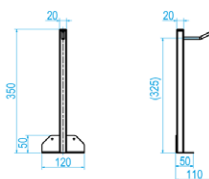
Hanger AK-AF5SL
