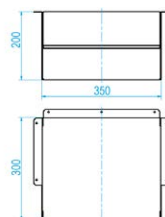
Box H-200, G-300, L-350 AK-ABG5S
